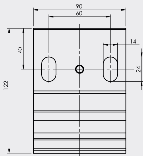
Monteringskonsol för kassett
