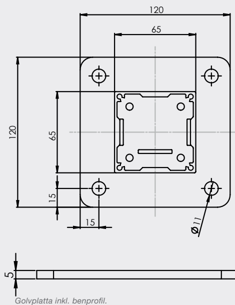
Golvplatta inkl. benprofil.
